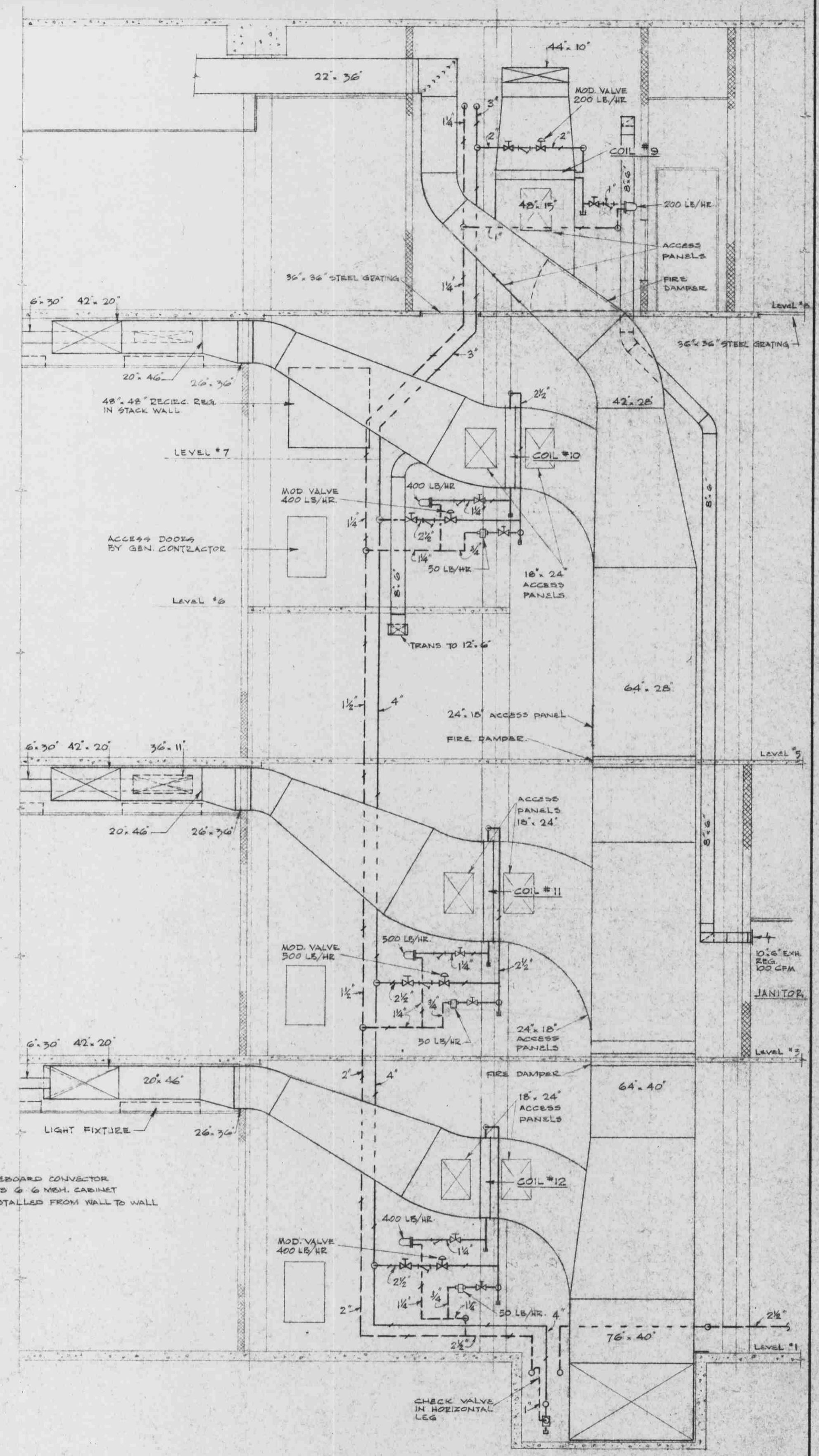
SECTION X-X SCALE: 1/8" = 1'-0"
