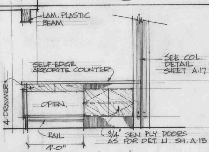
ELEVATION L
